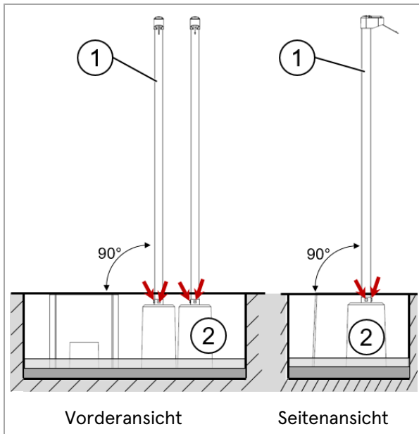
Abb. 39: KMS befestigen
