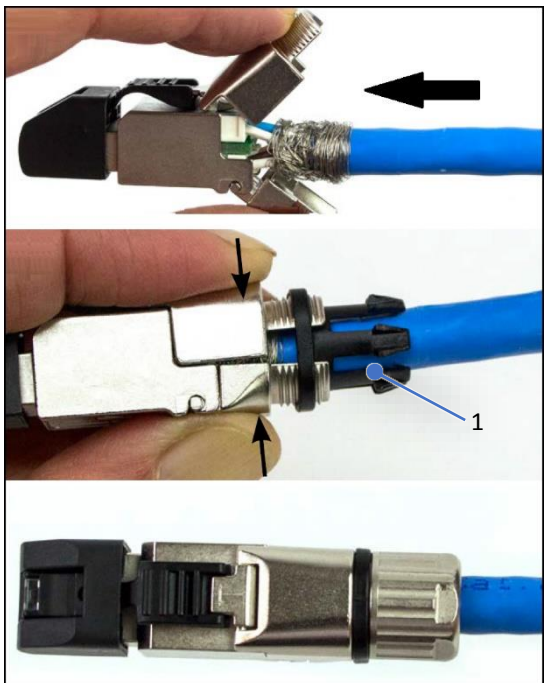
Abb. 31: RJ45 Steckverbindergehäuse
