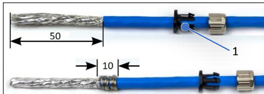
Abb. 27: Leitung abisolieren
