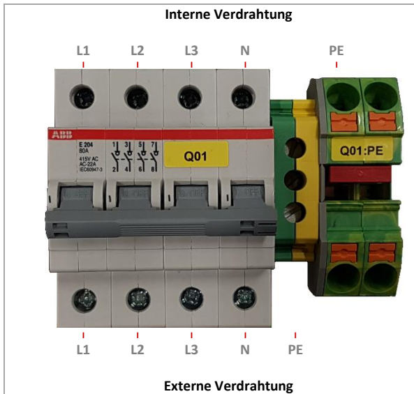
Abb. 22: Klemmleiste
