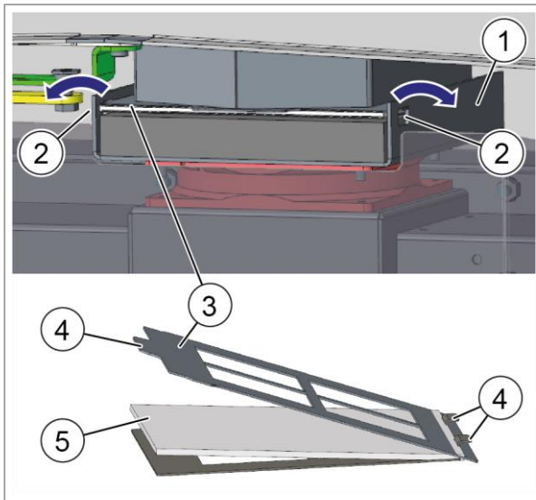
Abb. 44: Filtermatte – Luftauslass (oben)
