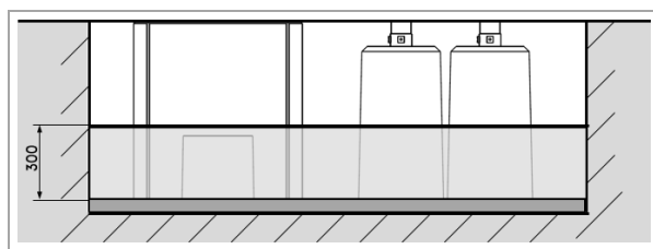
Abb. 40: Anfüllhöhe 300 mm
