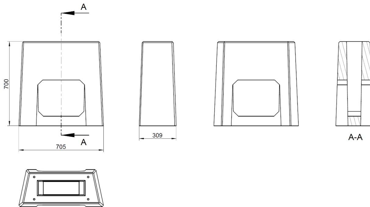
Konstruktionszeichnung des Beton-Sockels der Cito BM 240
