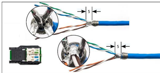
Abb. 28: Ladestück aufschieben
