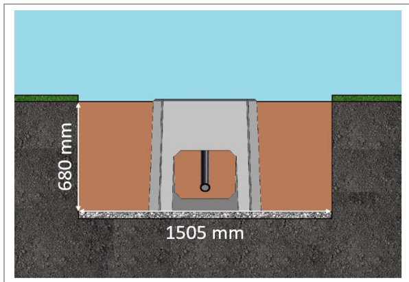
Abb. 16: Baugrube
