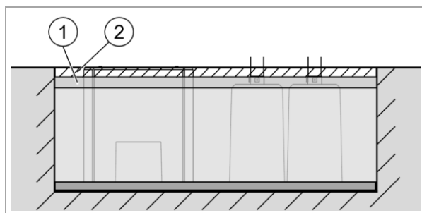
Abb. 42: Deckschicht einbringen
