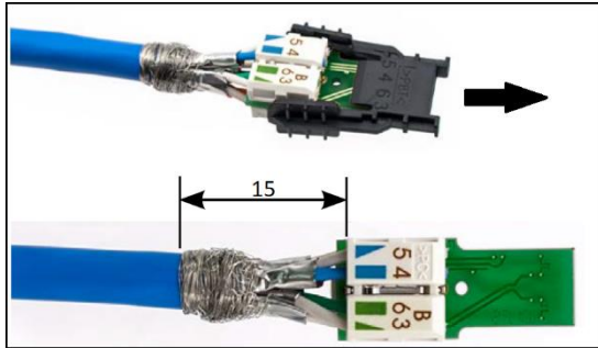
Abb. 30: Enden bündig abschneiden
