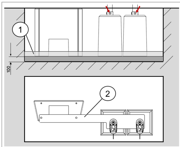
Abb. 38: Positionierhilfe montieren
