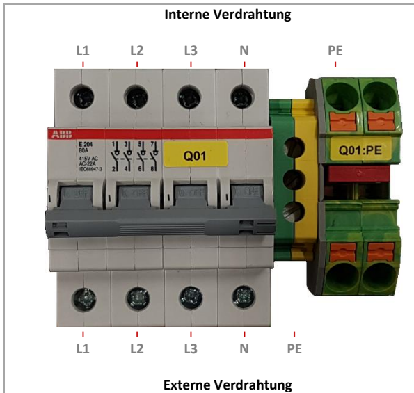
Abb. 22: Klemmleiste
