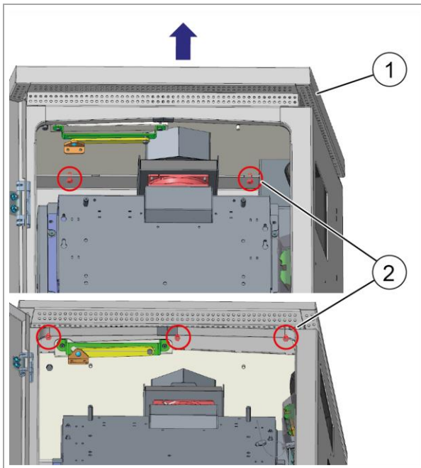
Abb. 5: Dach abnehmen
