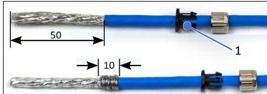
Abb. 27: Leitung abisolieren
