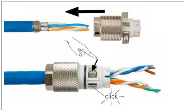
Abb. 24: Ladestück aufschieben
