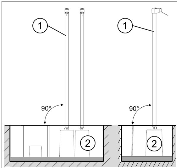
Abb. 37: KMS einsetzen
