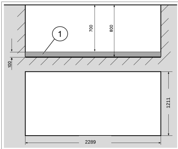
Abb. 35: Baugrube
