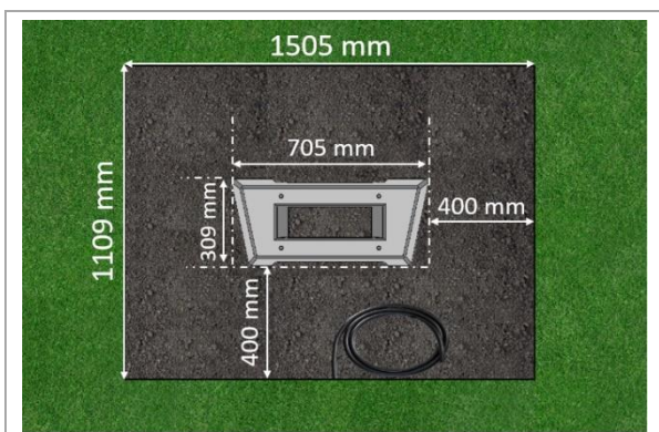
Abb. 15: Baugrube (Abmessungen)
