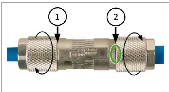
Abb. 26: Verschraubung schließen
