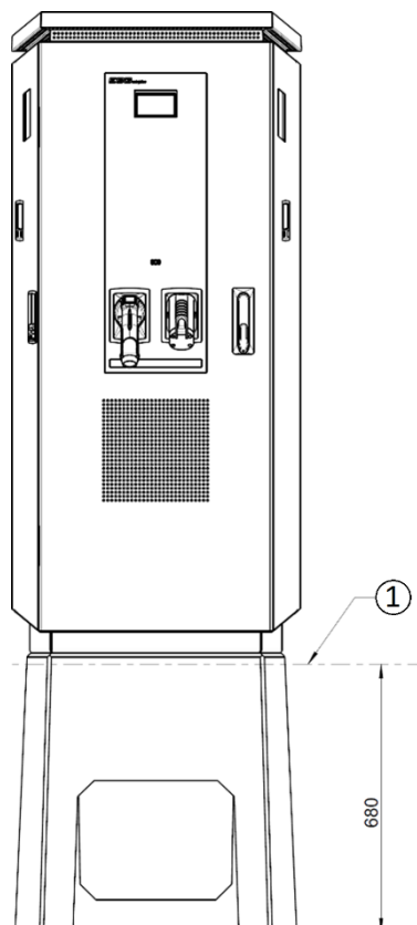
Konstruktionszeichnung des Ladesystems compleo® Cito BM 240
