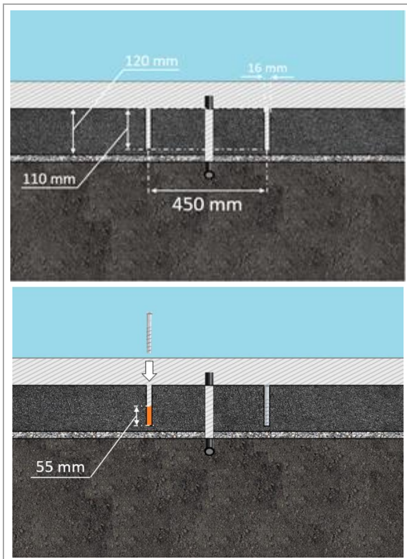
Abb. 12: Bohrlöcher
