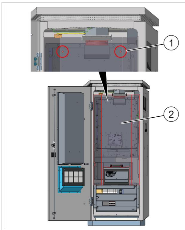
Abb. 4: Abdeckung vorne abnehmen
