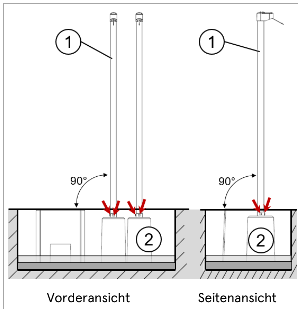
Abb. 39: KMS befestigen
