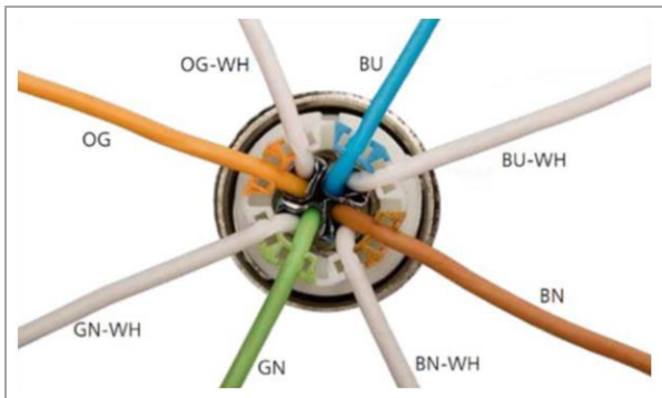
Abb. 25: Ladestück aufschrauben
