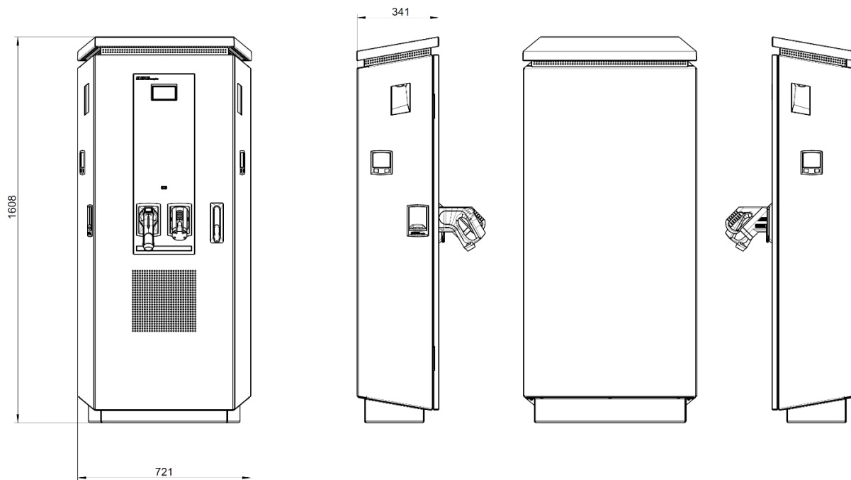
Konstruktionszeichnung des Ladesystems compleo® Cito BM 240
