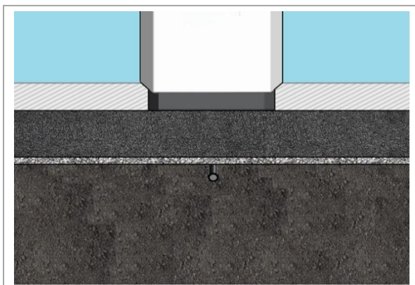
Abb. 13: Ladesystem befestigen
