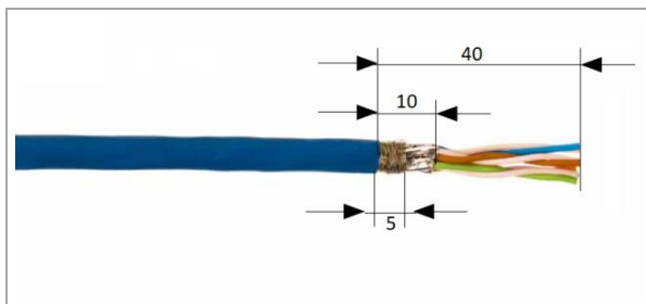
Abb. 23: Leitung abisolieren
