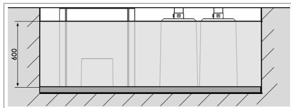
Abb. 41: Anfüllhöhe 600 mm
