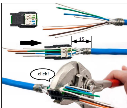
Abb. 29: Adern im Adernmanager befestigen
