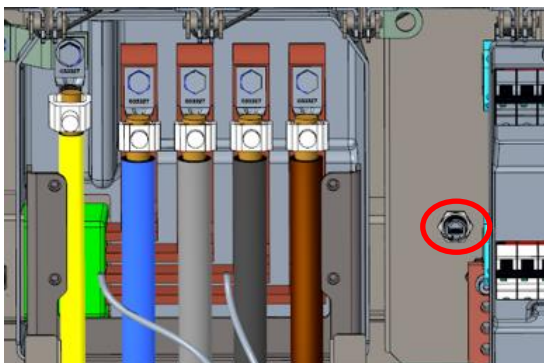
Abb. 32: Ladesystem verbinden
