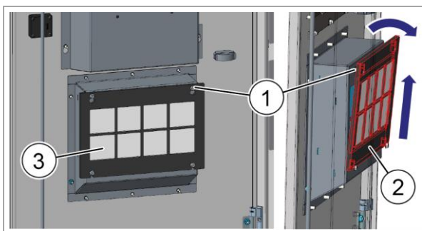
Abb. 45: Filtermatte – Lufteinlass (unten)
