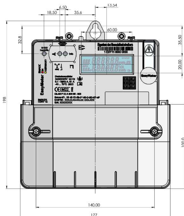
Drehstromzähler EasyM60®/ EasyM100® mit Klemmendeckel „60“
